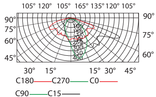
Intensité (cd/ 1000 lm) Diagramme Polaire
