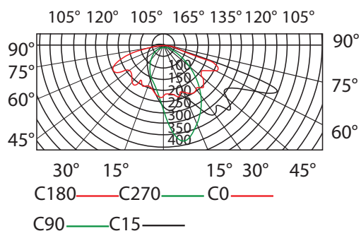
Intensité (cd/ 1000 lm) Diagramme Polaire
